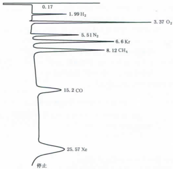
图 A.2 分子筛柱色谱图
